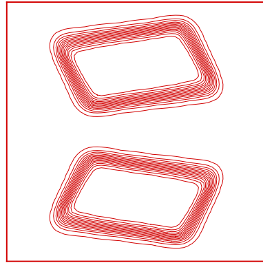
(b) 64^2 mesh
