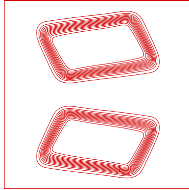
(d) 128^2 mesh
