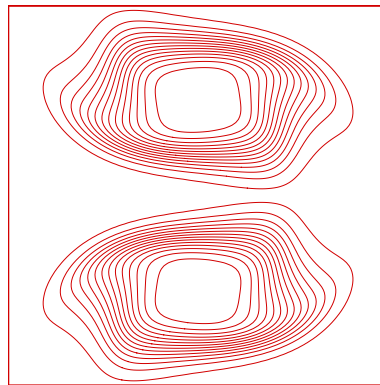
(d) 128^2 mesh
