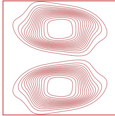
(b) 64^2 mesh
