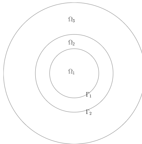
Fig. 1. Domain \Omega .
